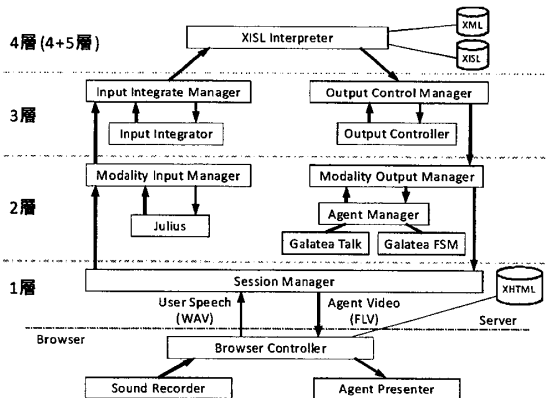
図3 6階層モデルに準拠したシステムのモジュール
