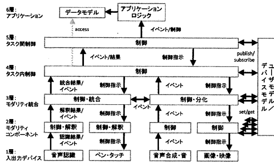
図2 MMI 6階層モデルのアーキテクチャ
