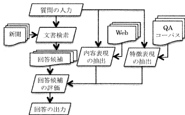
図 1 ベースライン手法の全体図
