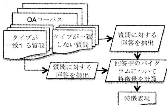
図 3 特徴表現の抽出手順
