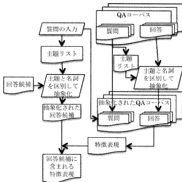
図4 主題を考慮した特徴表現による回答候補の評価
