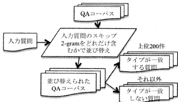
図 2 タイプが一致する質問の抽出手順
