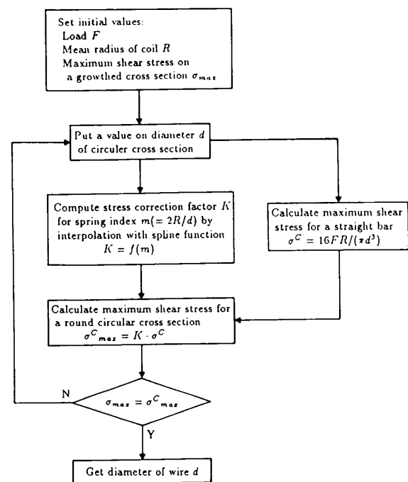
図 9 円形断面コイルばね素線直径 d の計算法
