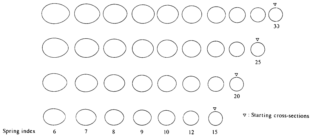
図 6 解析結果：ばね指数に対する素線断面形状
