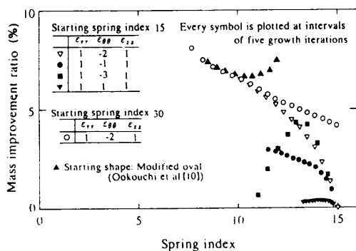
図 8 体積ひずみ発生則の検討結果
