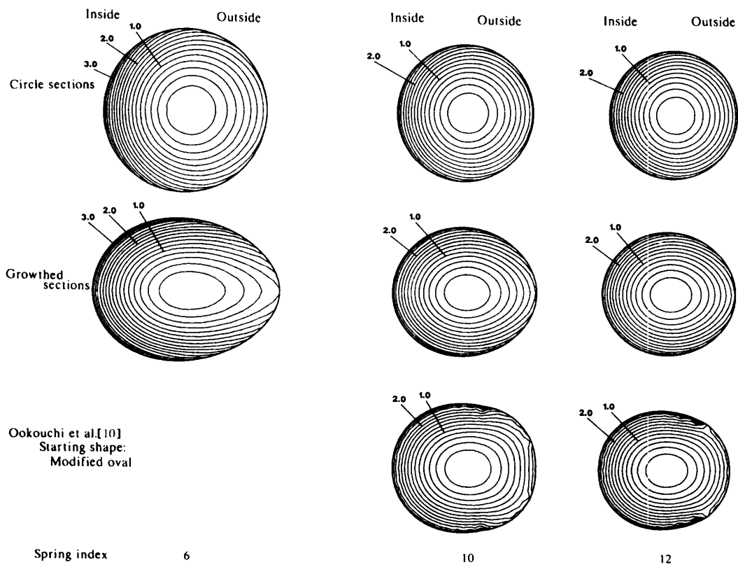
図 7 解析結果：ひずみエネルギー密度分布
