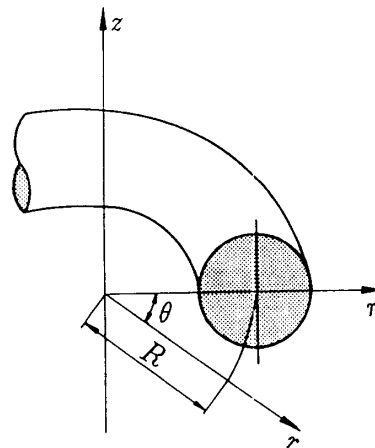
図2 円柱座標系によるコイル表記法
