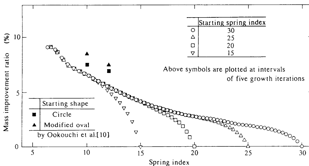
図5 解析結果: ばね指数に対する質量改善比
