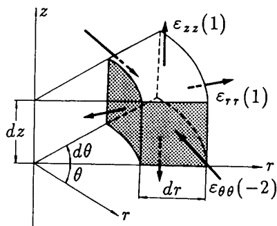
図3 体積ひずみ \epsilon_{ij}^B の発生則
