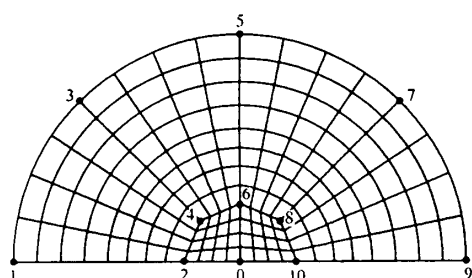
図4 素線断面の要素分割
