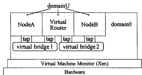
図2 Xenの内部ネットワーク構成例
