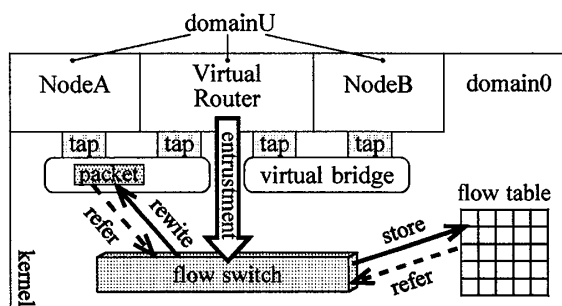
図4 フロースイッチの概要
