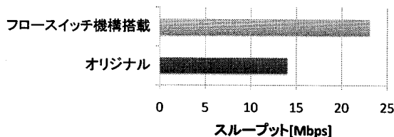
図 6 スループットの測定結果
