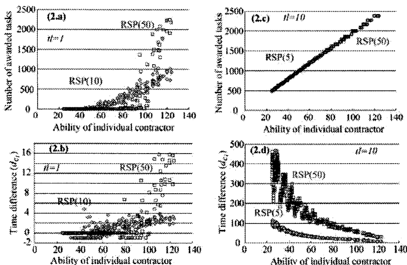
図2: RSP(n) を利用したときの総処理時間と入札値との差
