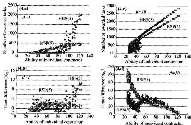
図4: HBS(5)を利用したときの総処理時間と入札値との差(RSP(5)との比較)
